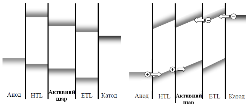
Рис.1.4 Енергетична схема шарів багатошарового OLED (а) і шарів багатошарового OLED у робочому режимі (б) [4].
