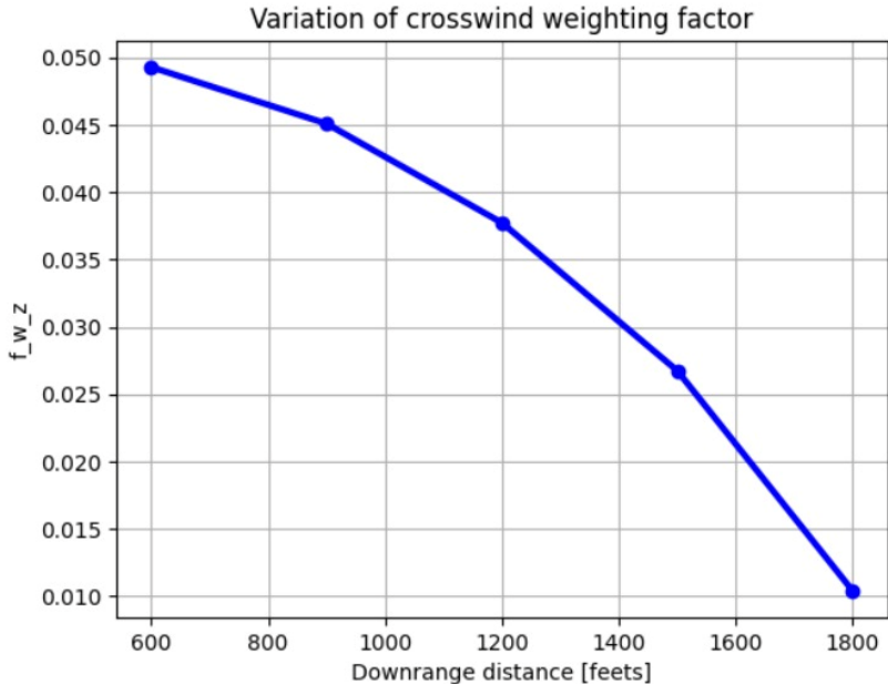
Рис. 1 Значення вагового коефіцієнту впливу вітру («чутливість») для патрону 30 Ball M2 в залежності від відстані від дульного зрізу.
