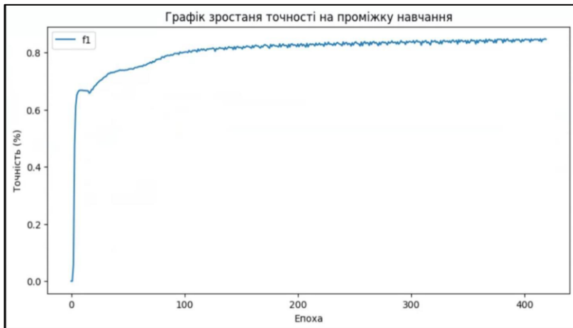
Рис 2. Графік зростання точності під час навчання моделі нейронні мережі на валідаційних даних
