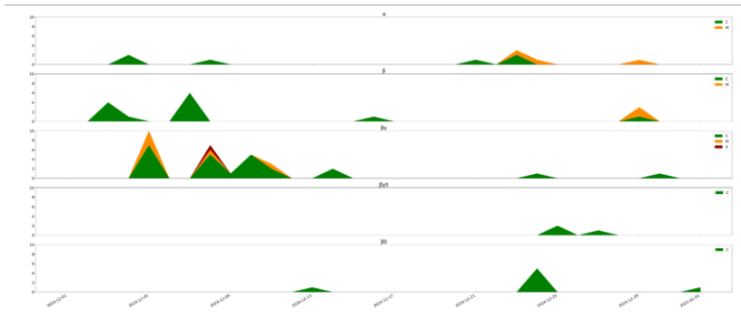
Рис. 1. Результат роботи програми, розробленої автором. Зміна кількості спалахів різних класів протягом грудня 2024
