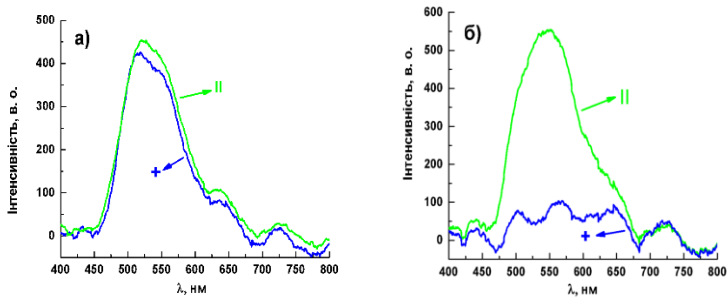
Рис.4 Спектри електролюмінесценції виміряні в схрещений (+) і паралельній (||) конфігурації поляризатора та зразка: а) OLED осадженого на підкладку розміщену перпендикулярно до потоку пари, б) OLED осадженого на підкладку розміщену під кутом 10^\circ до потоку пари.
