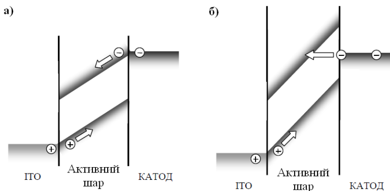
Рис.2 Енергетична схема OLED у робочому режимі (а) і з великим бар'єром для інжекції електронів у робочому режимі (б) [4].
